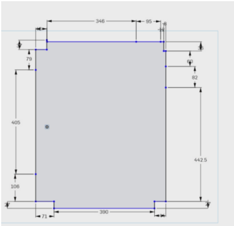
Grundriss Raum hinten links (Eingang ist oben
